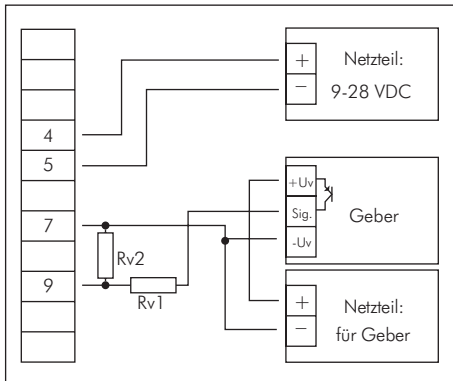
Anschluss eines Gebers (mit getr. Versorgung) mit PNP-Ausgang und externer Widerstandsbeschaltung
