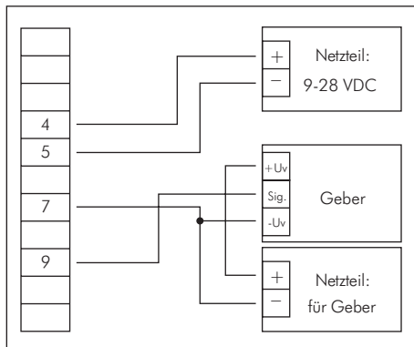
Anschluss eines Gebers (mit getr. Versorgung) mit TTL- oder PNP-Ausgang
